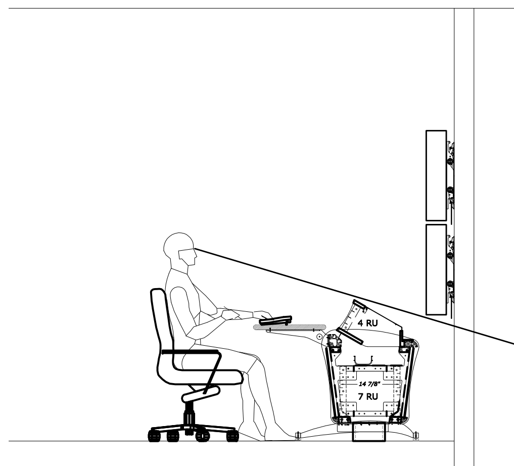
4 SECTION SCOREBOARD SCALE: 1/2" = 1'-0"
