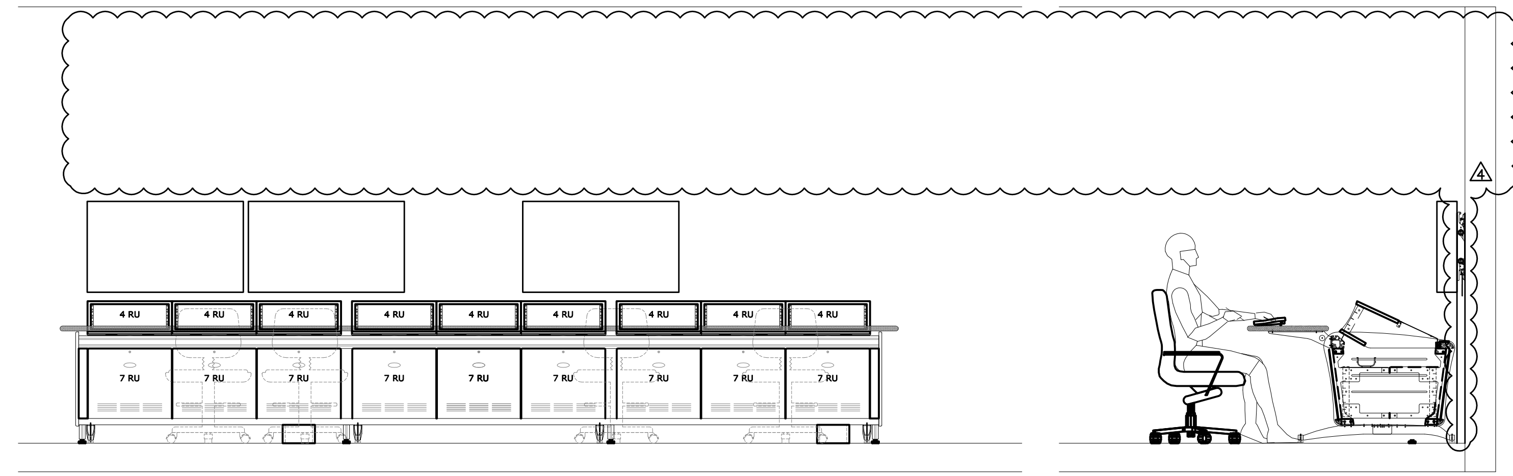
6 SECTION SCOREBOARD SCALE: 1/2" = 1'-0"
